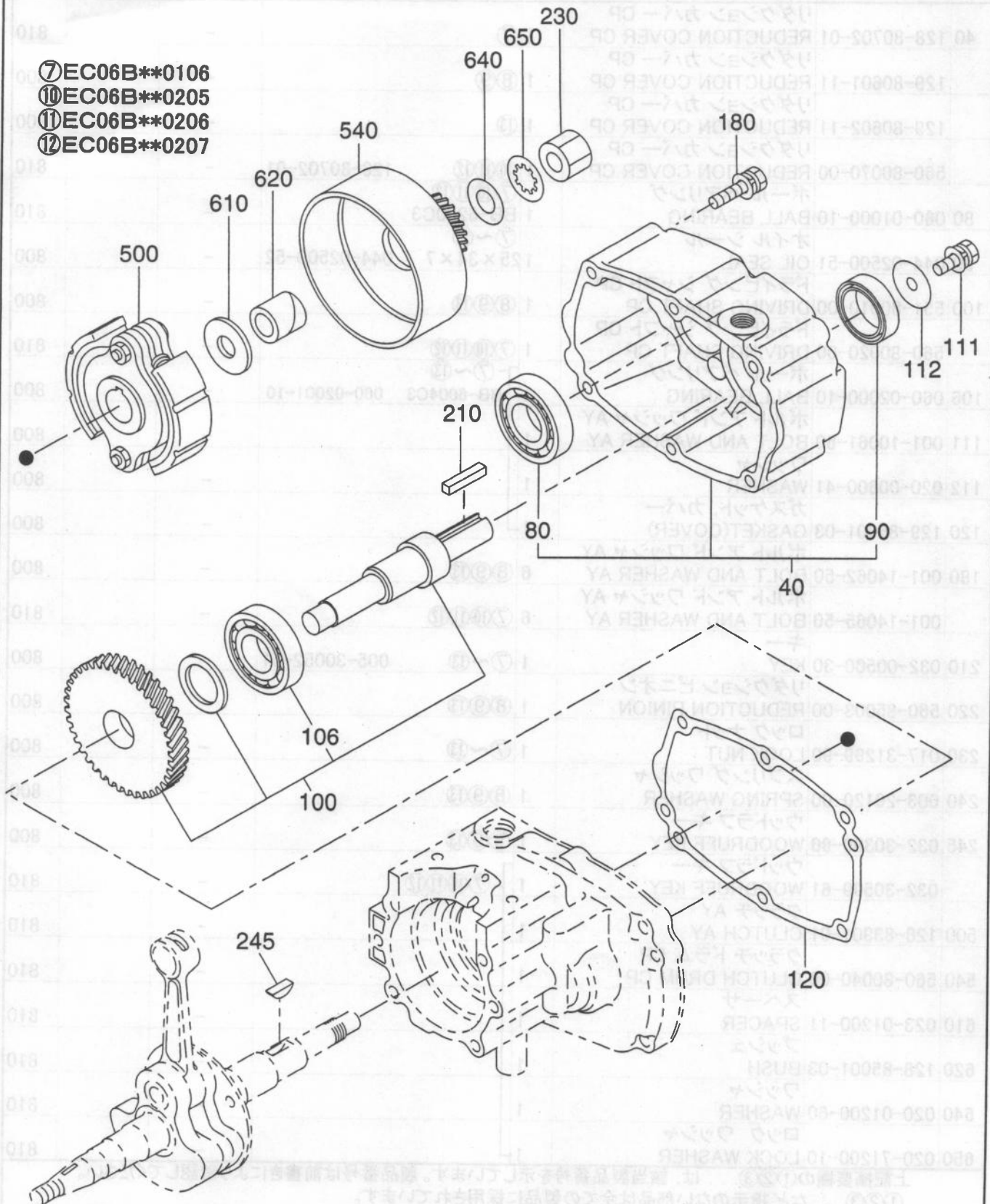
リダクション, クラッチ REDUCTION, CLUTCH
