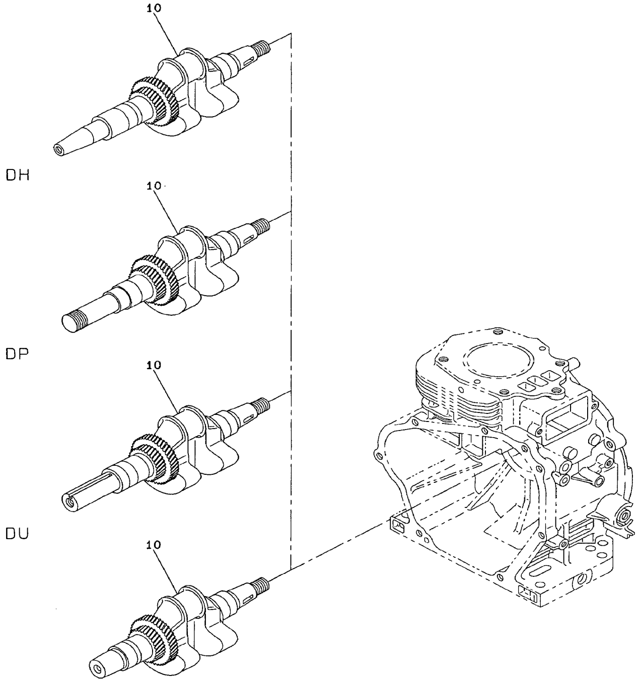
クランクシャフト CP. CRANKSHAFT CP.
