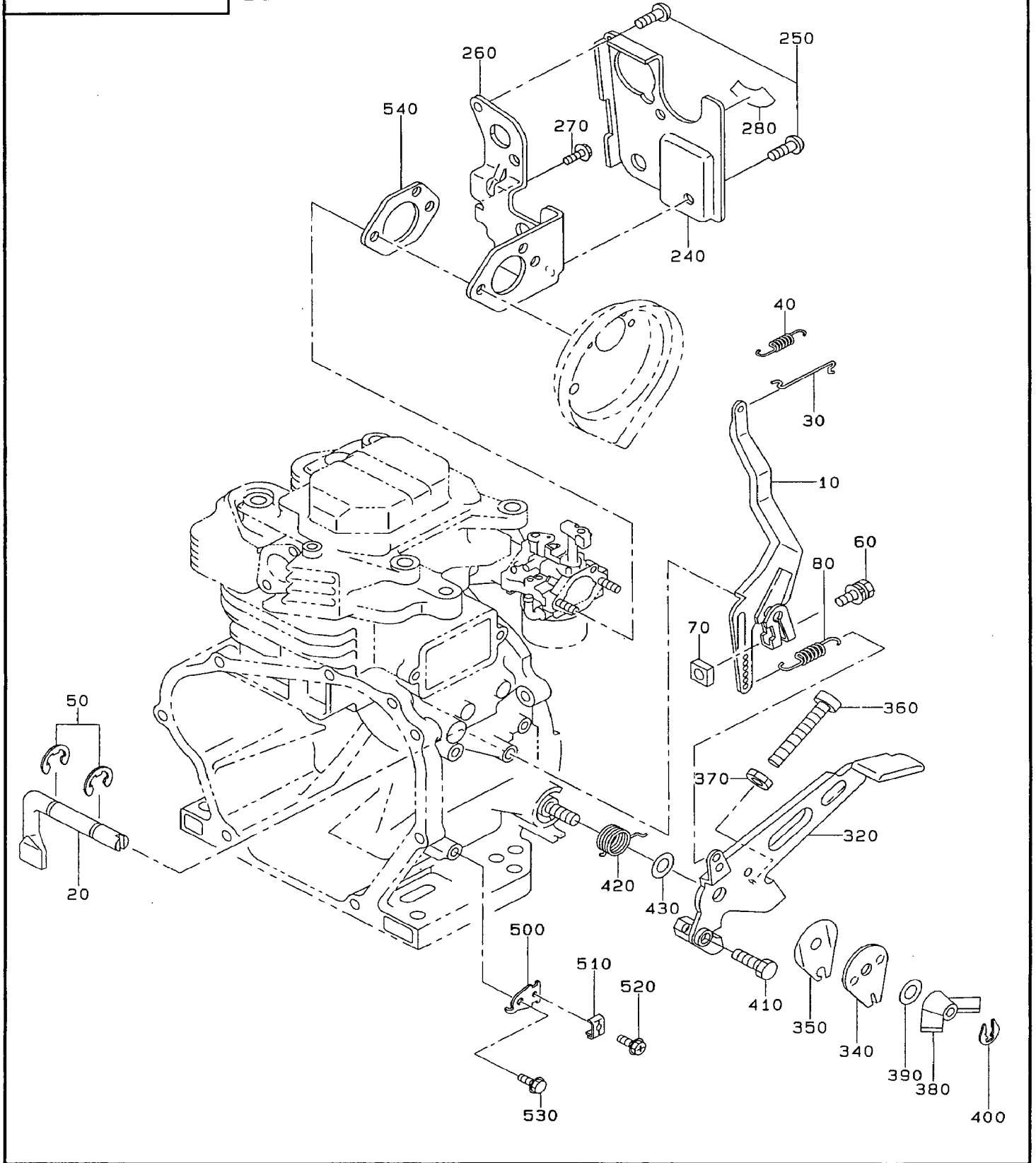
下索引仕様 LOWER CABLE CONTROL
